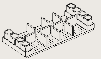
Inclut 10 séparateurs pour largeur de 1200 mm
